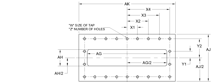
INLET/DISCH FLANGES
