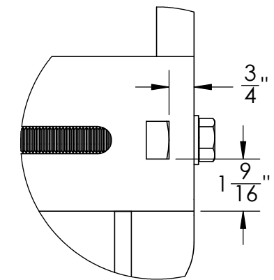
DETAIL B WELD NUT (4x TYP) SCALE 1 : 4
