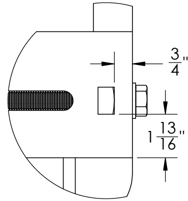
DETAIL B WELD NUT (4x TYP) SCALE 1 : 4
